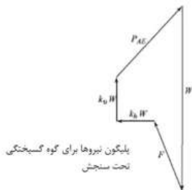
شکل پ ۹-۶ نحوه محاسبه نیروی محرک زلزله (معادله مونونوبه-اکابه)
