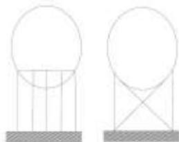
مخازن روی پایه با یا بدون مهاربندی R_{ii} = 3 یا 2
