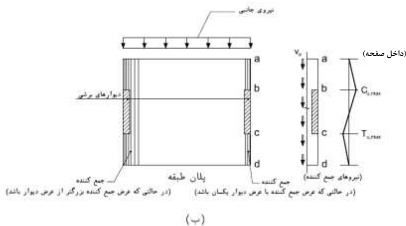
شکل پ ۳-۱ دیافراگم و اجزاء تشکیل دهنده آن
