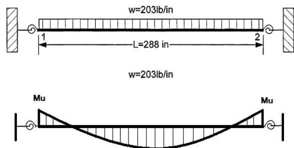
شکل (۳): مدل فنر دورانی جهت اتصال نیمه صلب
